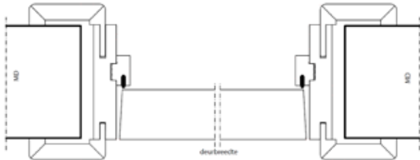
Horizontale doorsnede WoodFlex kozijn Section horizontale huisserie WoodFlex
