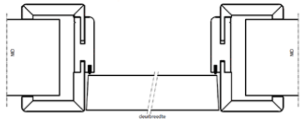
Horizontale doorsnede WoodFlex Style kozijn Section horizontale huisserie WoodFlex Style
