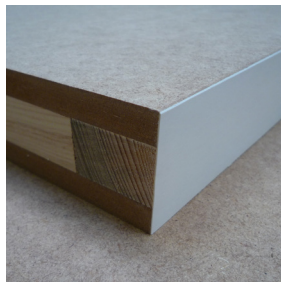
Detail body MDF 10 mm Détail body MDF 10 mm
